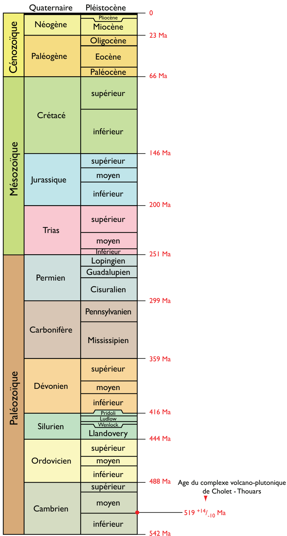
Echelle simplifiée des temps géologiques [d'après International Commission on stratigraphy, 2009]
